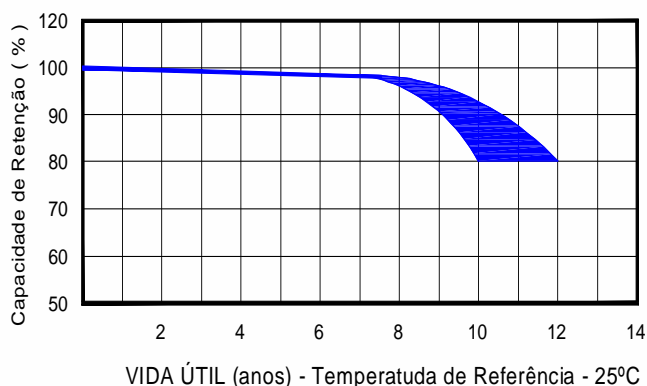
VIDA ÚTIL EM FLUTUAÇÃO - MODELOS DE 33 a 250 Ah
