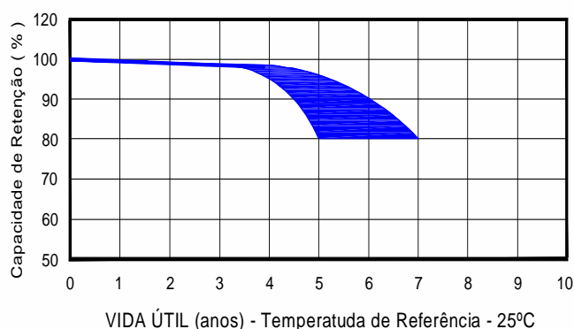
VIDA ÚTIL EM FLUTUAÇÃO - MODELOS DE 5 a 26 Ah
